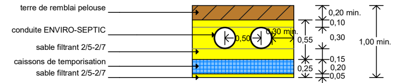
COUPE TRANSVERSALE
